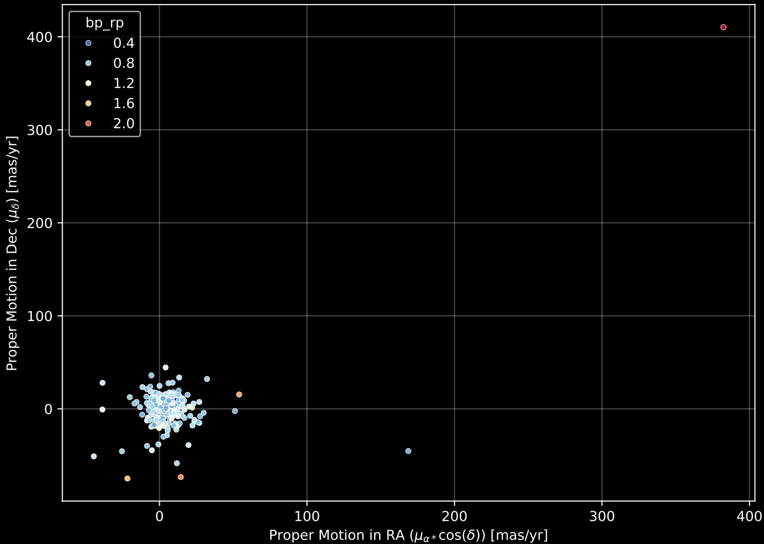
GALAH DR4 Field: [586] Proper Motion Diagram (n= 300)
