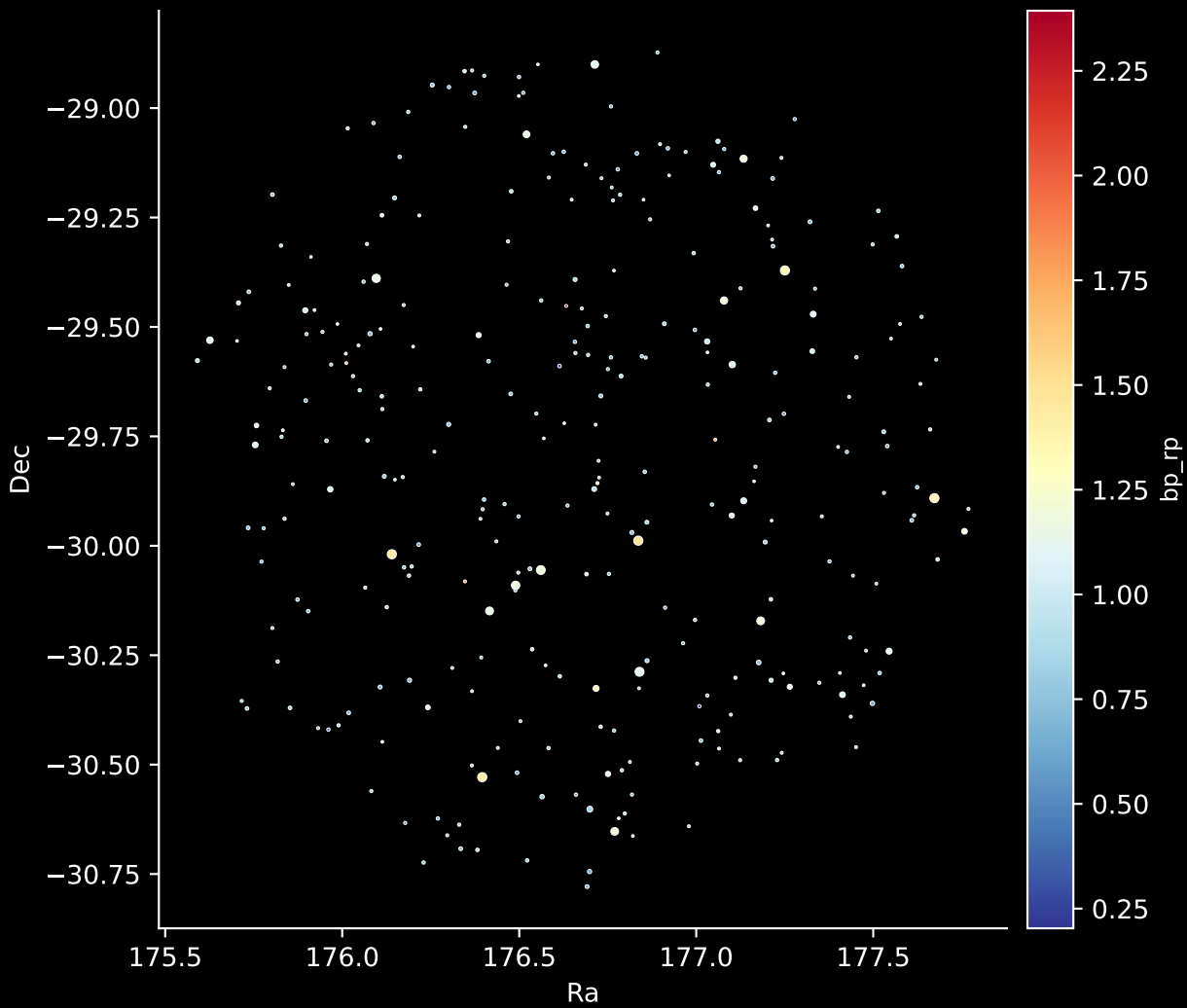
GALAH DR4 Field: [586] Stars: 300
