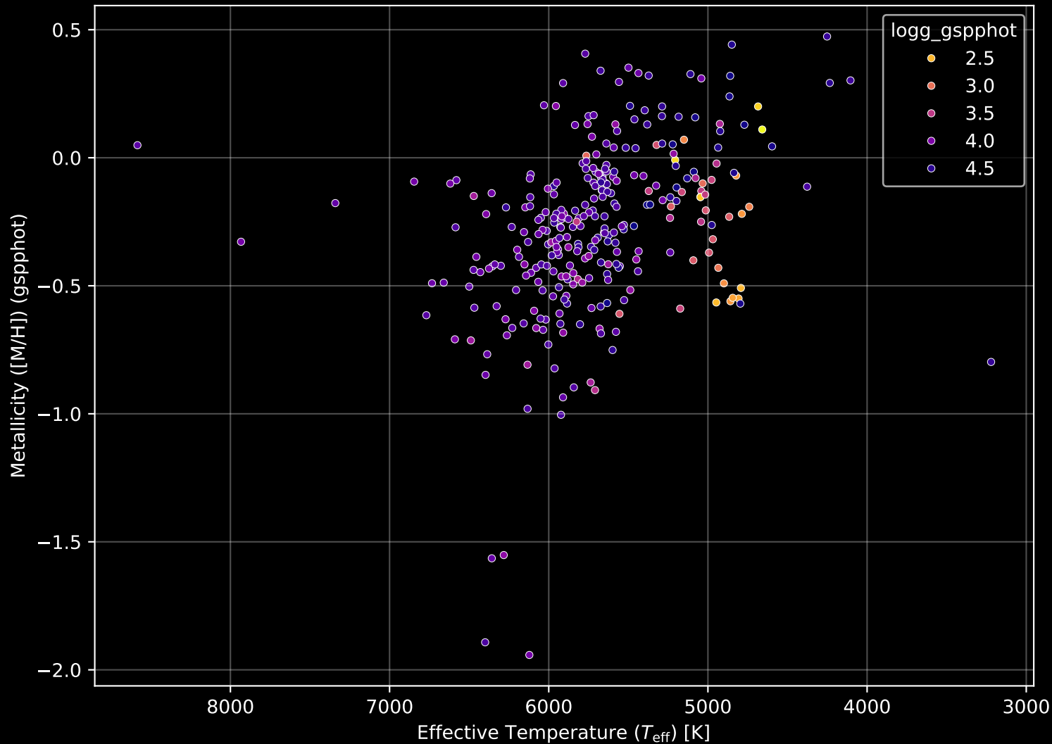
GALAH DR4 Field: [586] Stellar Population Parameters (n= 300)
