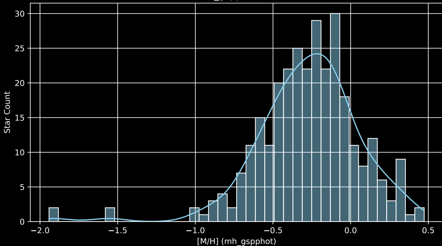
GALAH DR4 Field: [586] [M/H] (mh_gspphot) (n= 300)
