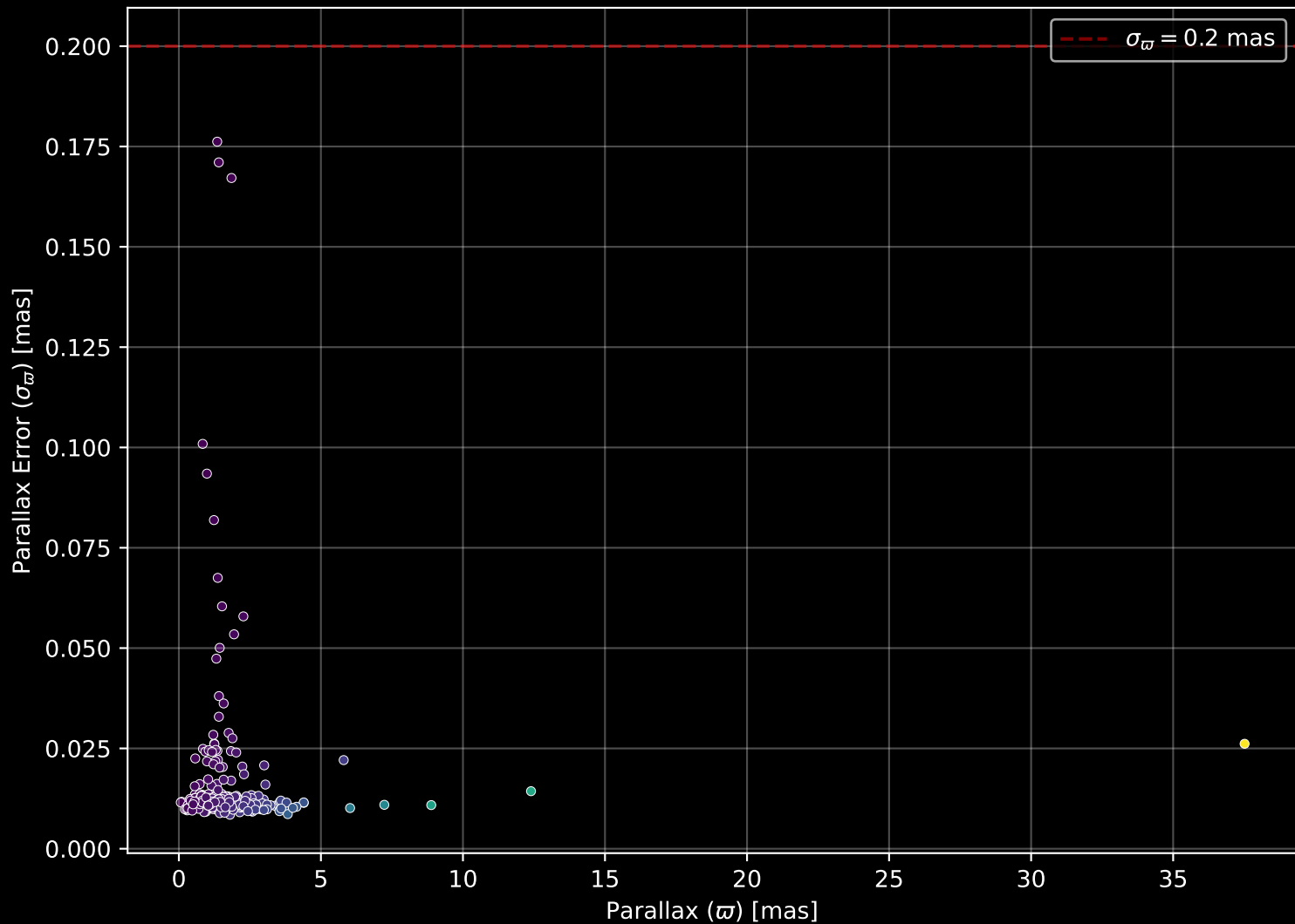
GALAH DR4 Field: [586] Parallax Quality (n= 300)
